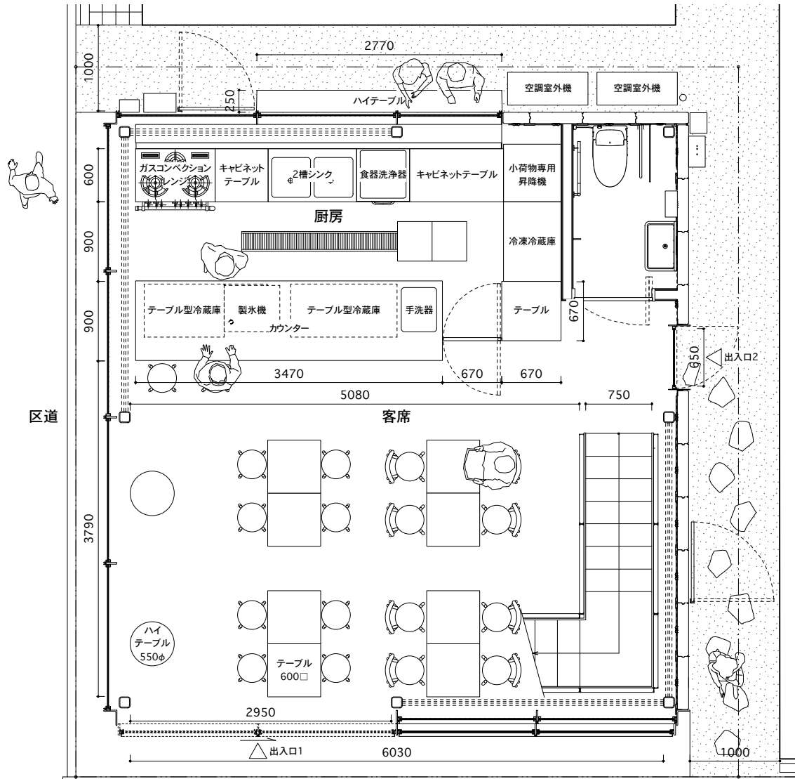
Kitchen Studio SUIBA レイアウト参考図 S=1:100(A4)
